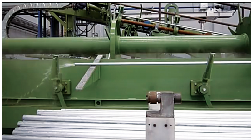
Dây chuyền sản xuất Ống thép mạ kẽm Galvanized Steel Pipe Production Line
