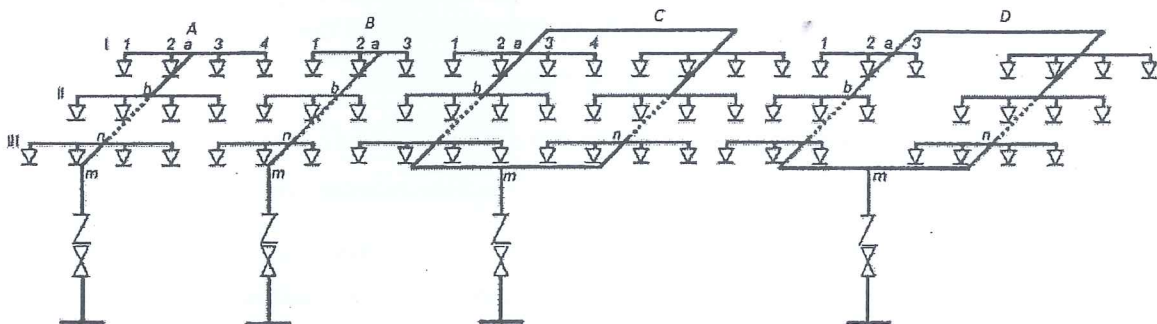
Hình B.1 - Các sơ đồ mạng lưới phân phối của hệ thống chữa cháy Sprinkler hoặc Drencher
