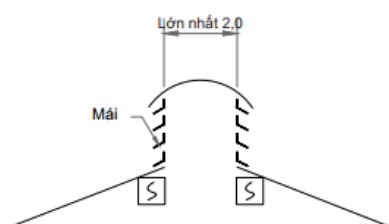
(h) Lỗ thông của dầm góc hẹp
