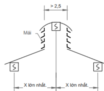
(i) Lỗ thông của dầm góc rộng
