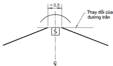
(f) Dầm nóc có thông gió
